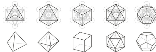
Tetraeder Würfel/Hexaeder Dodekaeder Oktaeder Icosaeder
